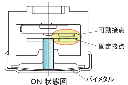
動作原理図
